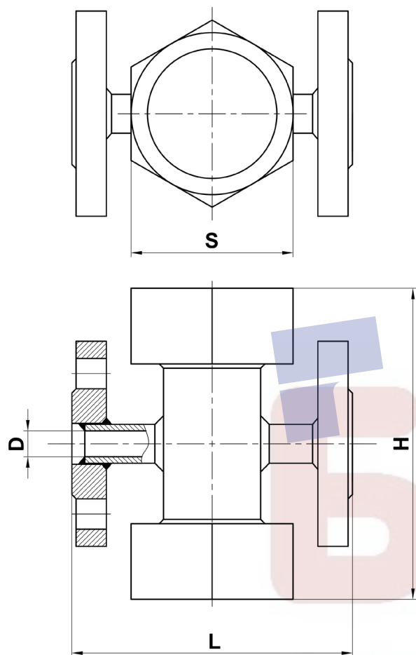
ИЗ33, ИЗ35 (фланцевое исполнение)
