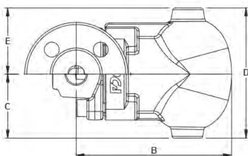
Линейная конструкция
