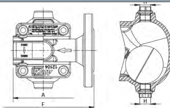
Линейная конструкция
